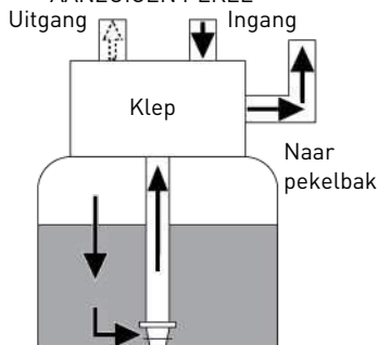
C5 AANZUIGEN PEKEL
